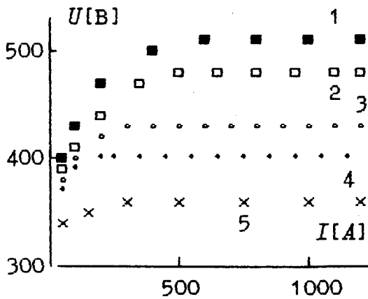
Рис. I.9 Сильноточный (а) и высоковольтный (б) режимы [64-66]. а. 1- Ag , p = 2 \cdot 10^{-2} тор, 1- B = 670 Гс, 2- B = 1360 Гс, 3- B = 1800 Гс, 4, 5- N_2 , H_2 , б. He p = 1 \cdot 10^{-3} тор, 1- B = 1360 Гс, 2- B = 910 Гс, 3- B = 670 Гс,
