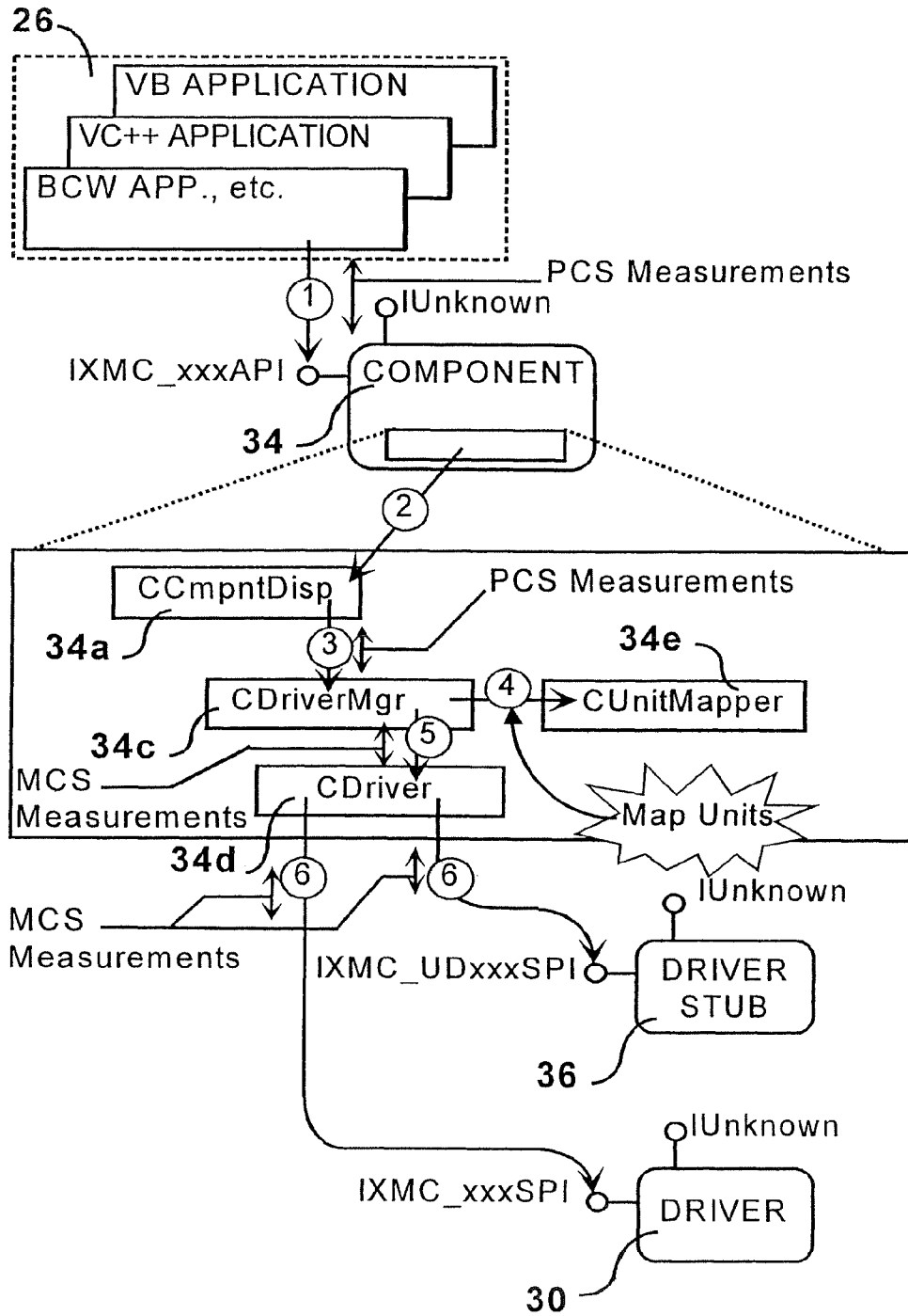
FIG. 6 Scenario-Map - Unit Mapping
