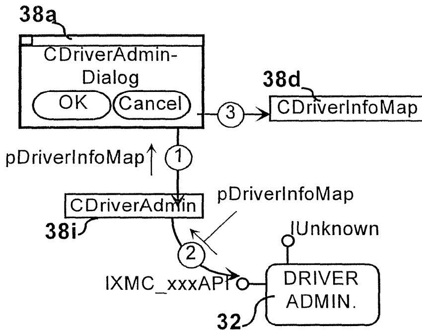
FIG. 54 Scenario-Map - Main Dialog Init.
