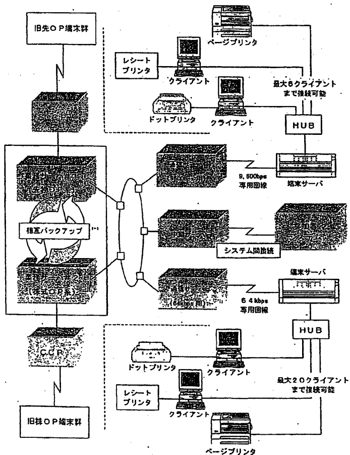
1-1 システム構成図
