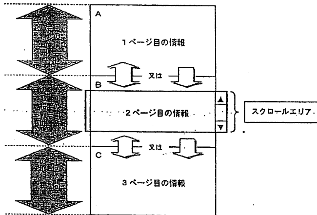
※頁単位での問合せ（問合せ応答情報取得）例
