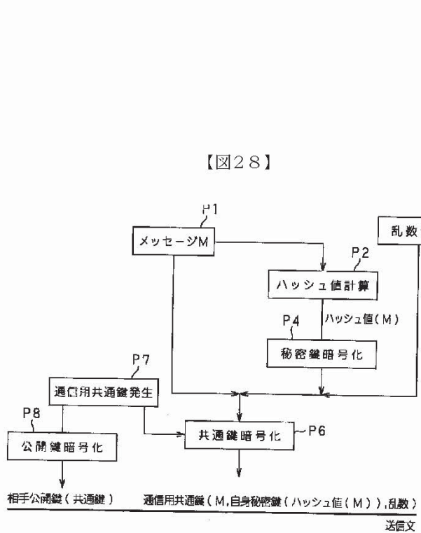
使用情報返却時のユーザ端末のフローチャート
