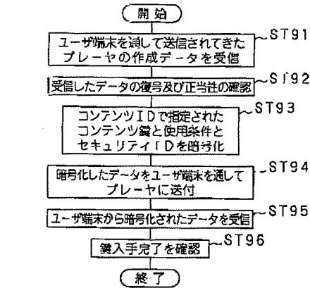
コンテンツ鍵・使用条件入手時の管理センタのプロトコルチャート
