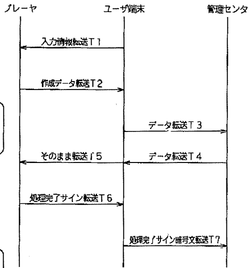
ポイント購入時のシーケンス
